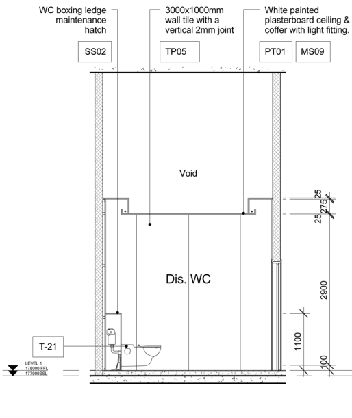
Elevation 21 SCALE: 1 : 50
