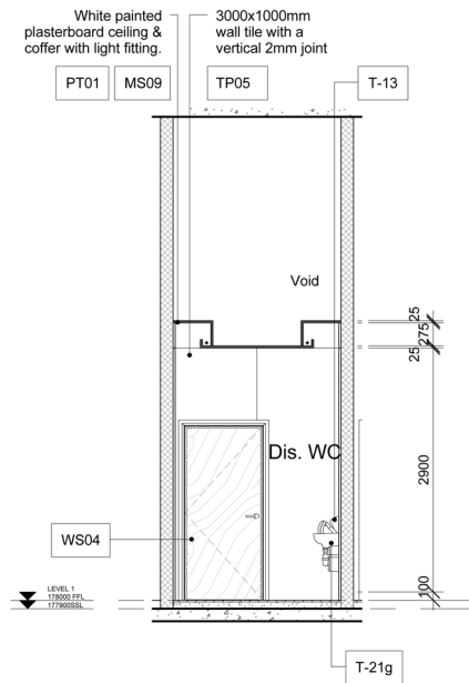
Elevation 22 SCALE: 1 : 50
